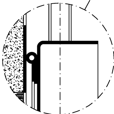
Scheiteldichtung
